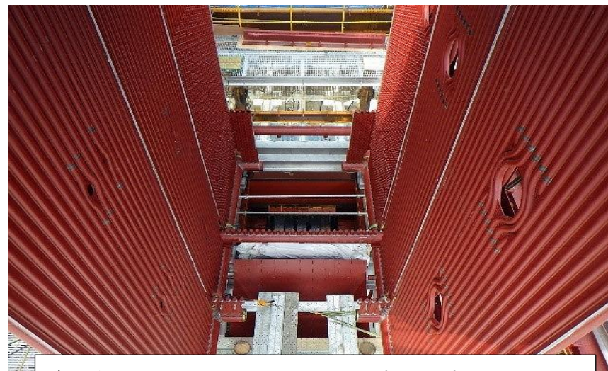
(8) 熱回収施設：ボイラパネル据付中
