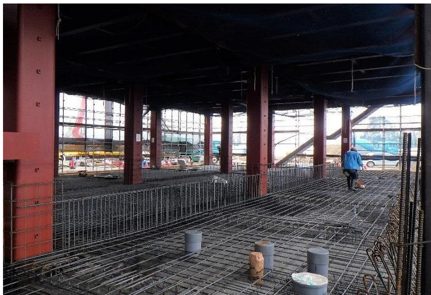
(3) 熱回収施設：ランプウェイ基礎パイルスタッド施工中
