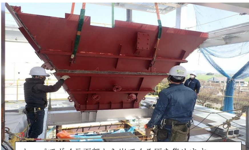
(7) 熱回収施設：ボイラホップ据付中
