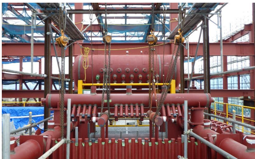
(7) 熱回収施設：ボイラドラム据付
