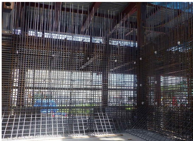
(3) リサイクル施設：2F スラブ施工
