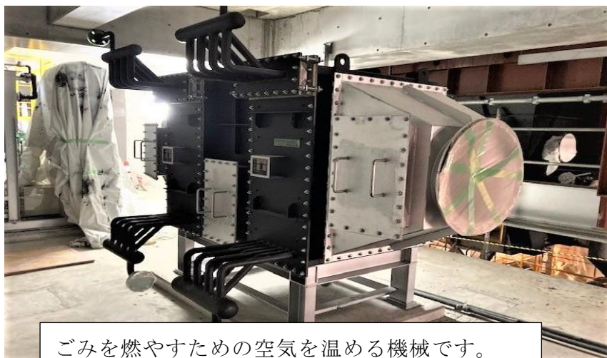
(7) 熱回収施設：蒸気式空気予熱器据付
