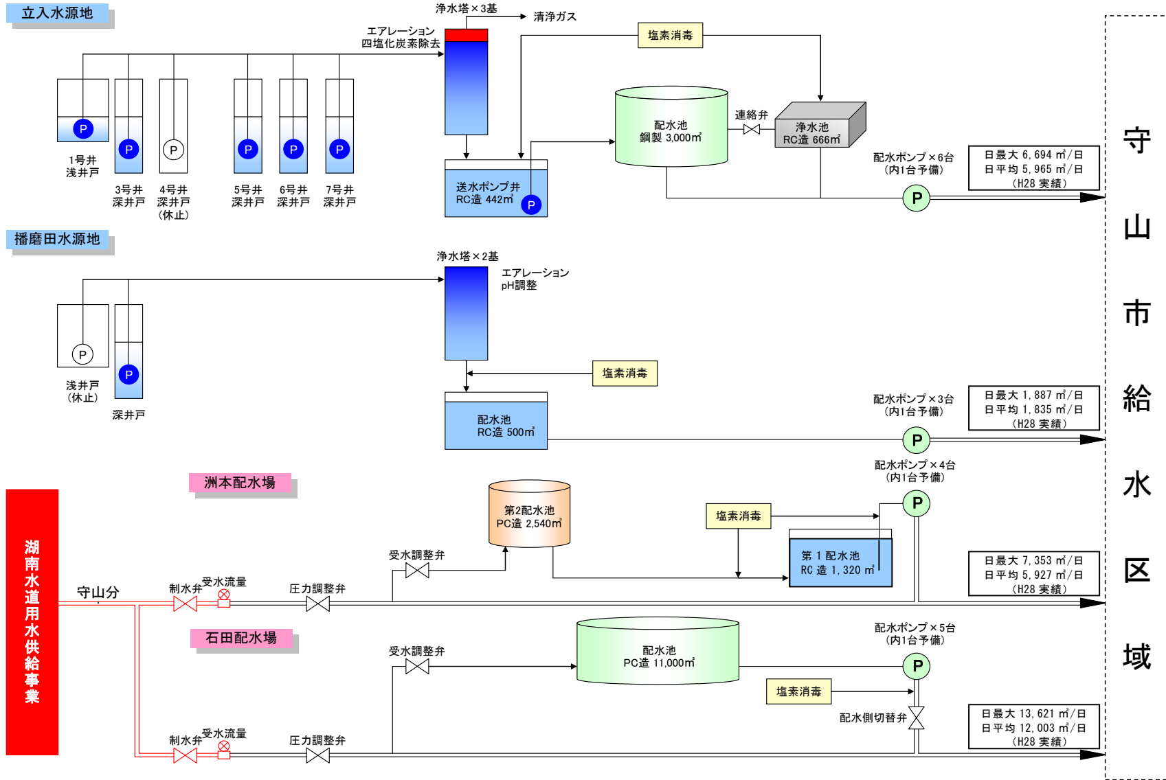
施設系統
