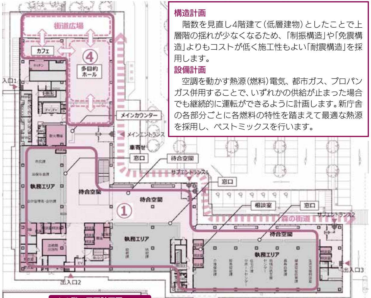
▲1階 平面計画図
