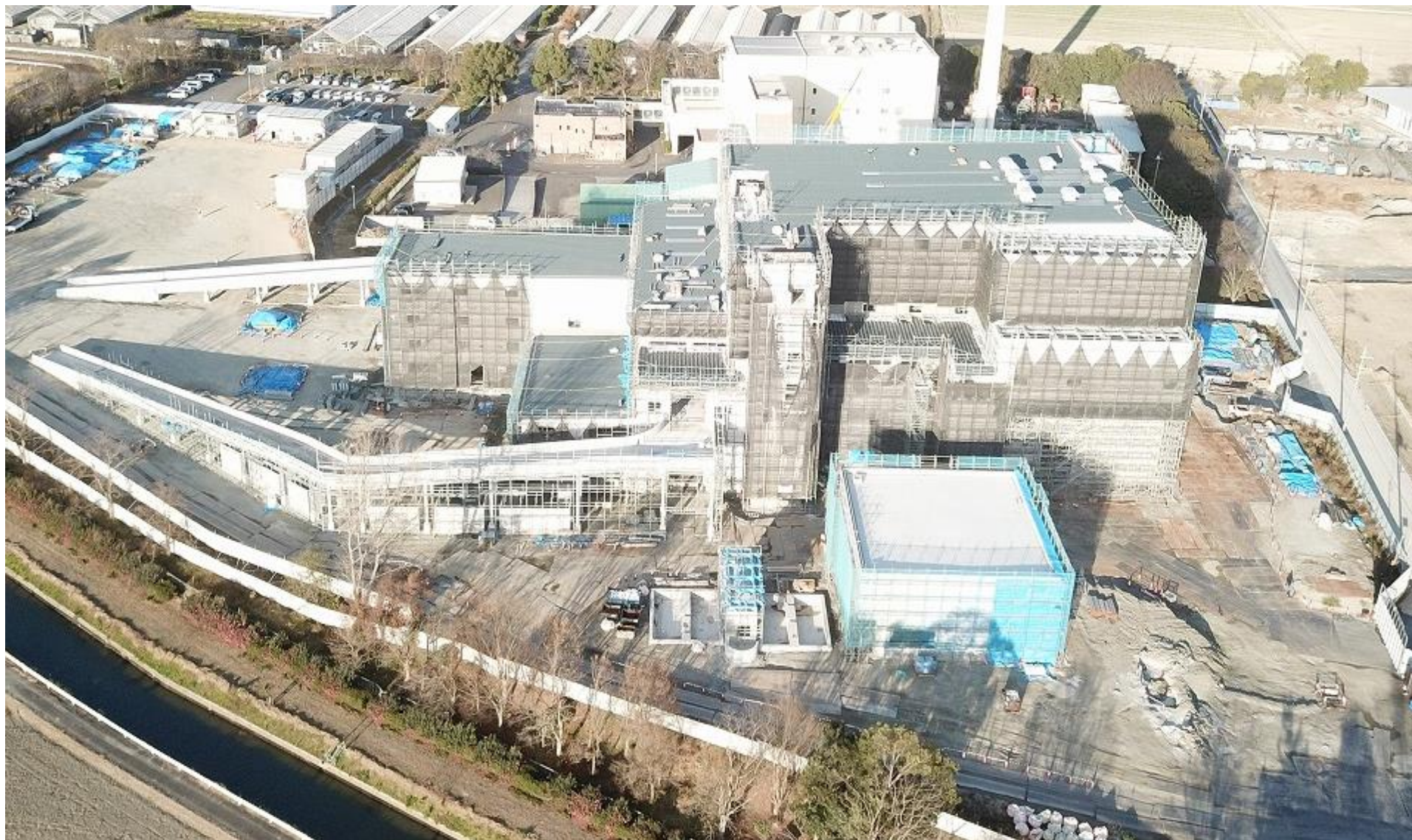
令和2年12月（2020年12月）の工事状況 12月25日撮影
