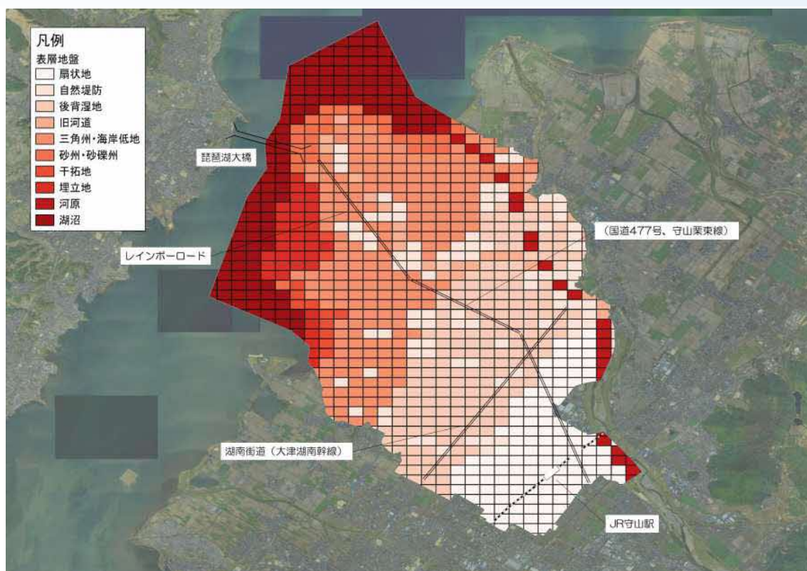
図 2.1-9 微地形区分図
