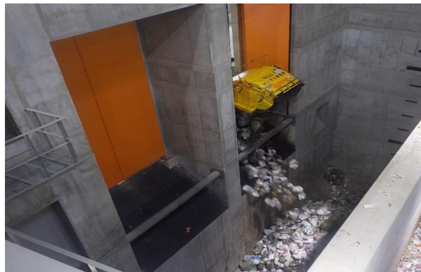
(2) 熱回収施設：ごみ受入れ開始（受入ピット）
