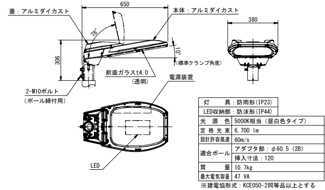
電源ユニット内蔵形
