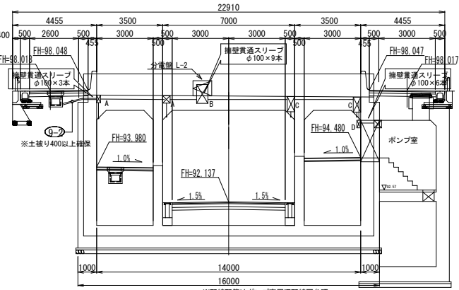
アンダーバス起点側断面図 S=1/100
