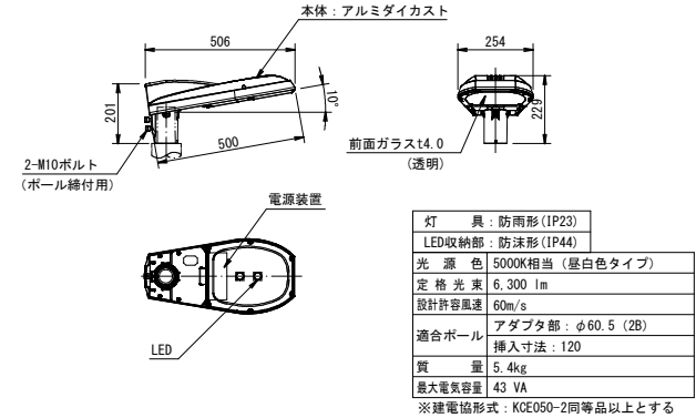
道路照明器具参考図 1: 10 (A1) 1: 20 (A3) 電源ユニット内蔵形
