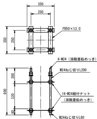
アンカーボルト詳細図 1: 10 (A1) 1: 20 (A3)
