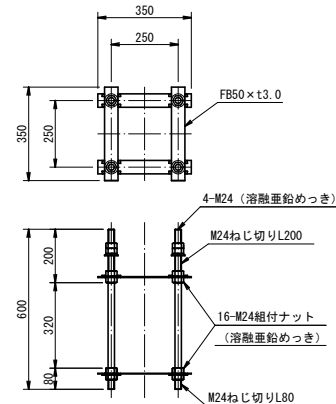
アンカーボルト詳細図
