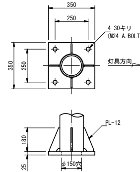
ベースプレート詳細図
