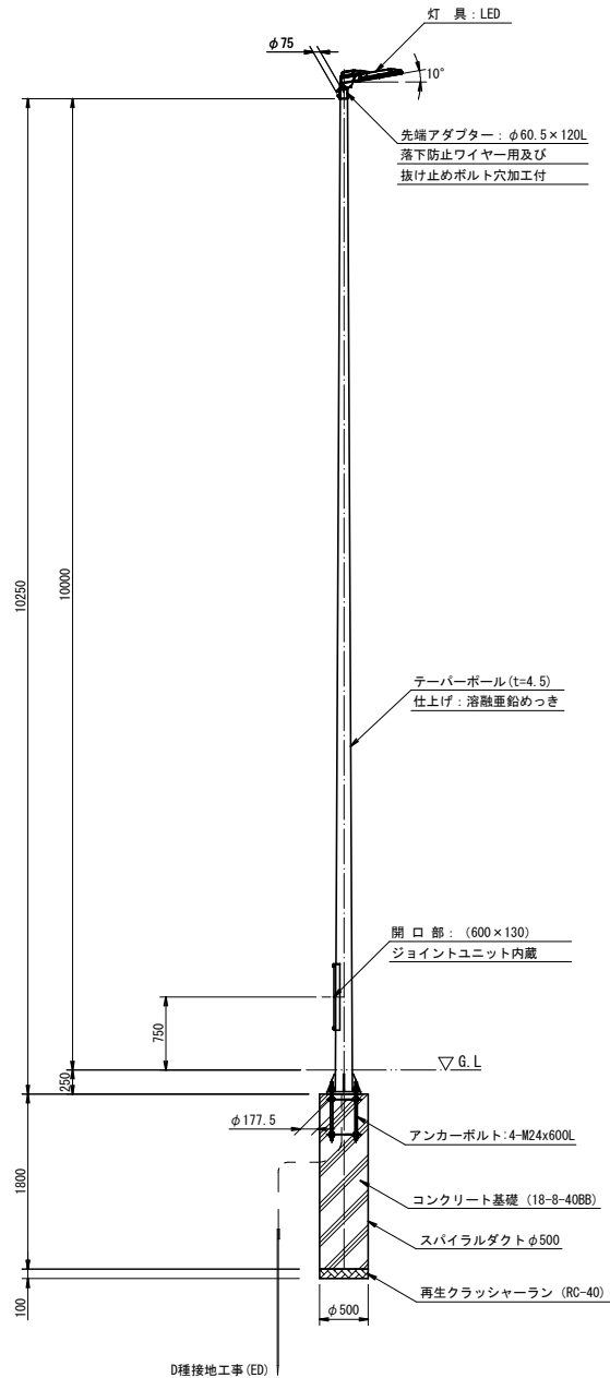
照明柱姿図
