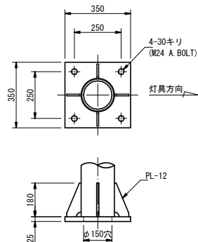
ベースプレート詳細図 1: 10 (A1) 1: 20 (A3)
