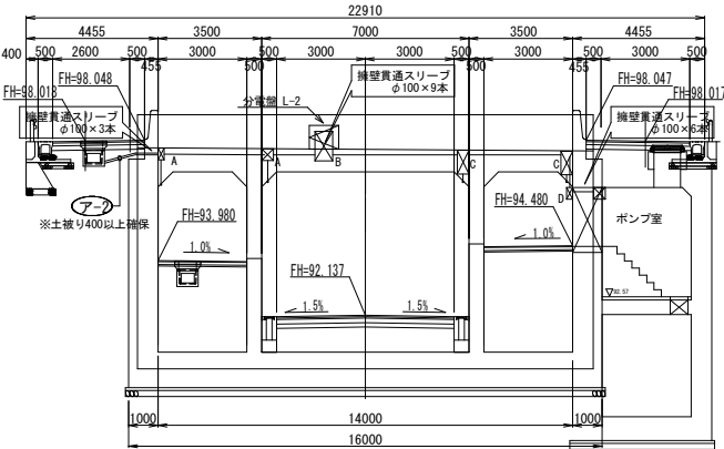
アンダーパス起点側断面図 S=1/100
