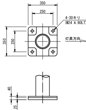
ベースプレート詳細図 1: 10 (A1) 1: 20 (A3)
